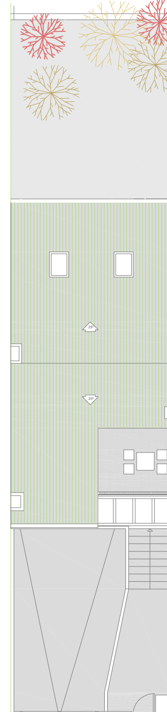
PLANTA CUBIERTA
