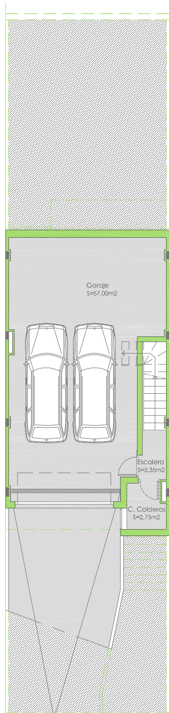
PLANTA SÓTANO
