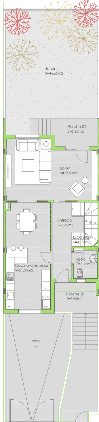
PLANTA BAJA
