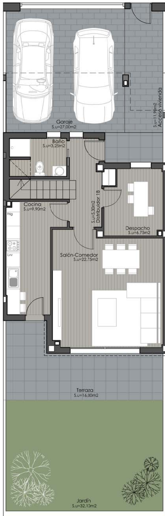
PLANTA BAJA
